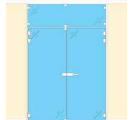
⑱ DUBBELE GLASDEUR met doorlopend vast bovenstuk
