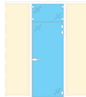
⑰ ENKELE GLASDEUR met doorlopend vast bovenstuk
