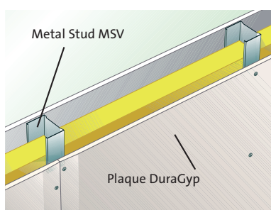
Ossature simple avec une couche de plaques DuraGyp
