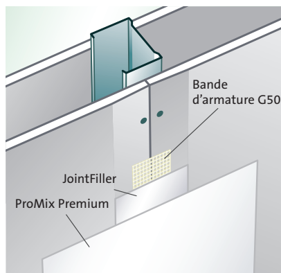
Technique de jointoiment ABA avec bande d'armature autocollante G50.
