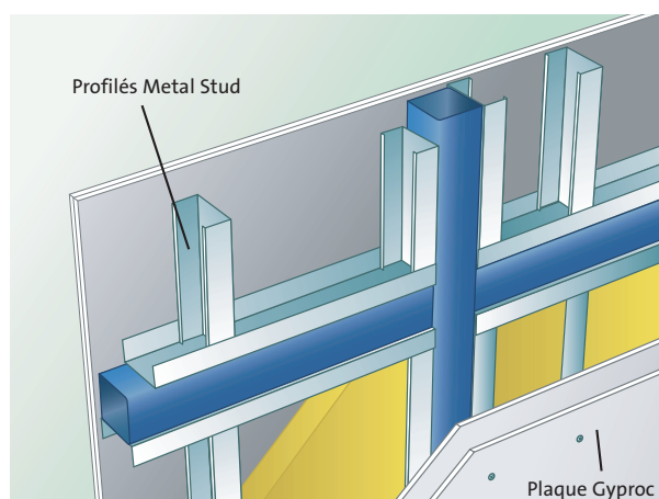
Structure portante en profilés tubulaires intégrée dans une cloison Metal Stud à ossature simple.
