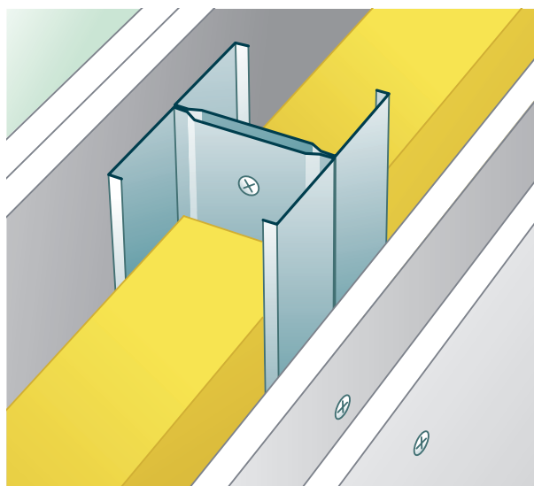
Doublages des montants
