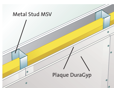
Ossature simple avec double couche de plaques DuraGyp
