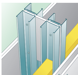
Ossature double et montants accouplés doubles.
