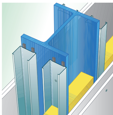
Fixation d'une cloison Metal Stud à double ossature à une colonne en acier.
