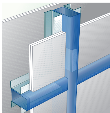
Cloison Metal Stud intégrée à la structure.
