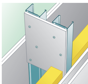
Ossature double et montants accouplés simples.
