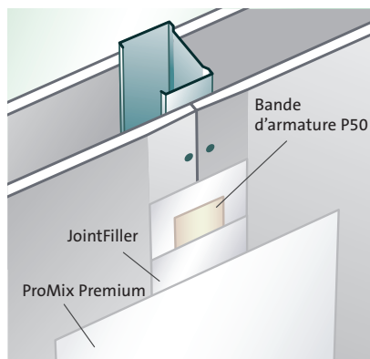
Technique de jointoiment ABA avec bande d'armature en papier P50.
