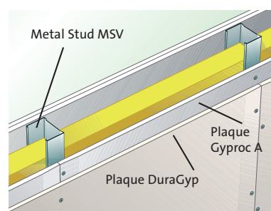
Ossature simple avec double couche de plaques combinées
