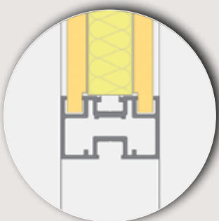
volle uitvoering
