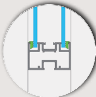
dubbele beglazing
