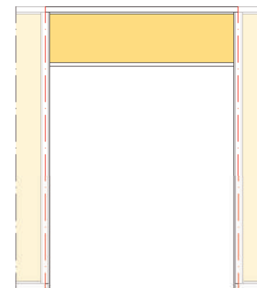
㉑ VOL BOVENLICHT voor dubbele deur
