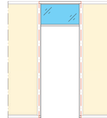
⑱ BEGLAASD BOVENLICHT enkel glas, voor enkele deur
