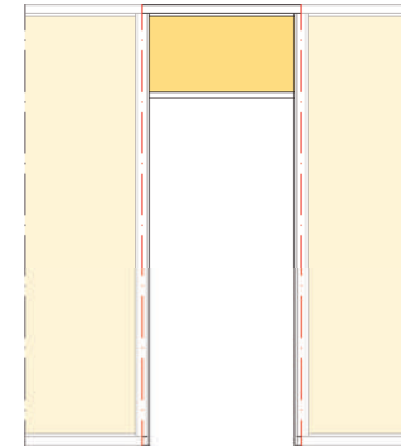
⑰ VOL BOVENLICHT voor enkele deur
